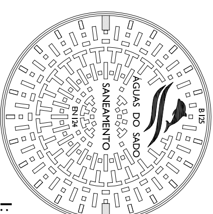
TAMPA TIPO
